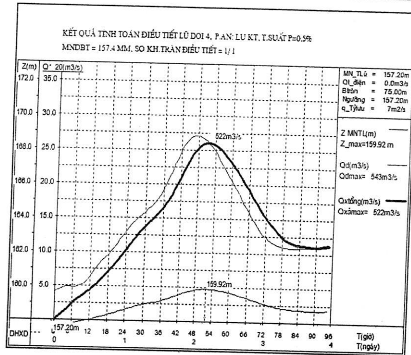
Hình PL 0-2: Quá trình lũ đến và xả lũ kiểm tra tần suất P = 0,5%
