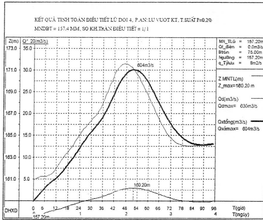
Hình PL 0-3: Quá trình lũ đến và xả lũ vượt tần suất P = 0,2%
