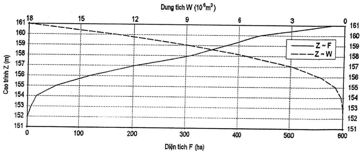
Hình PL 0: Biểu đồ quan hệ đường đặc tính lòng hồ chứa
