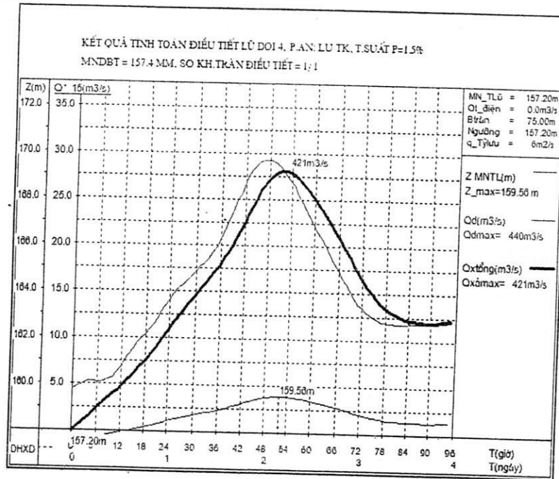
Hình PL 0-1: Quá trình lũ đến và xả lũ thiết kế tần suất P = 1,5%
