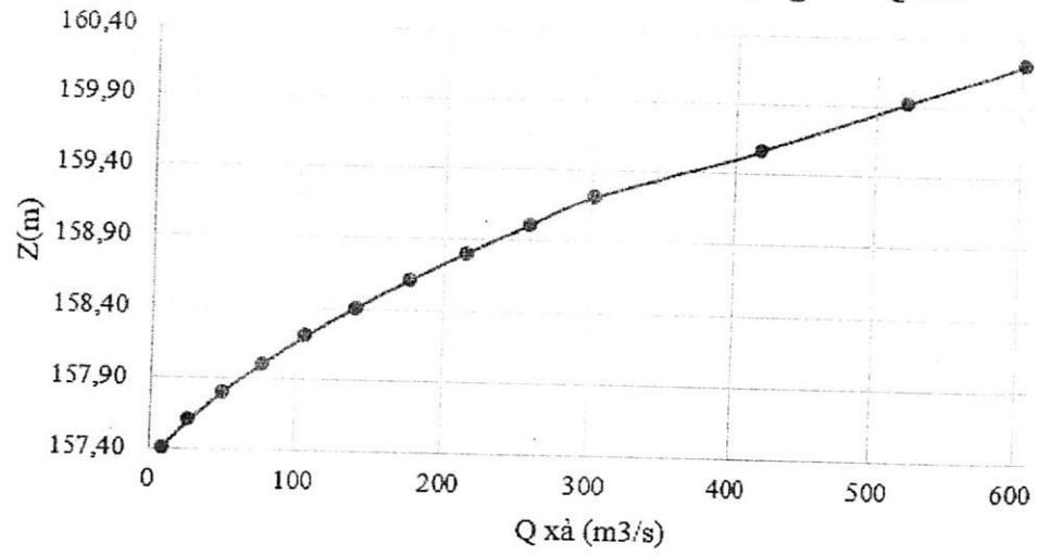
Hình PL 0: Quan hệ mực nước hồ và lưu lượng xả ( Z \sim Q )
